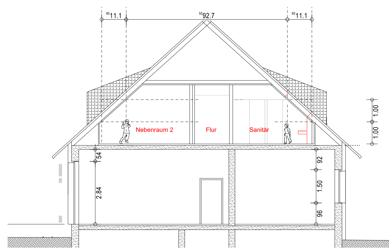
SCHNITT 2 Sanitär - Nebenraum 2
