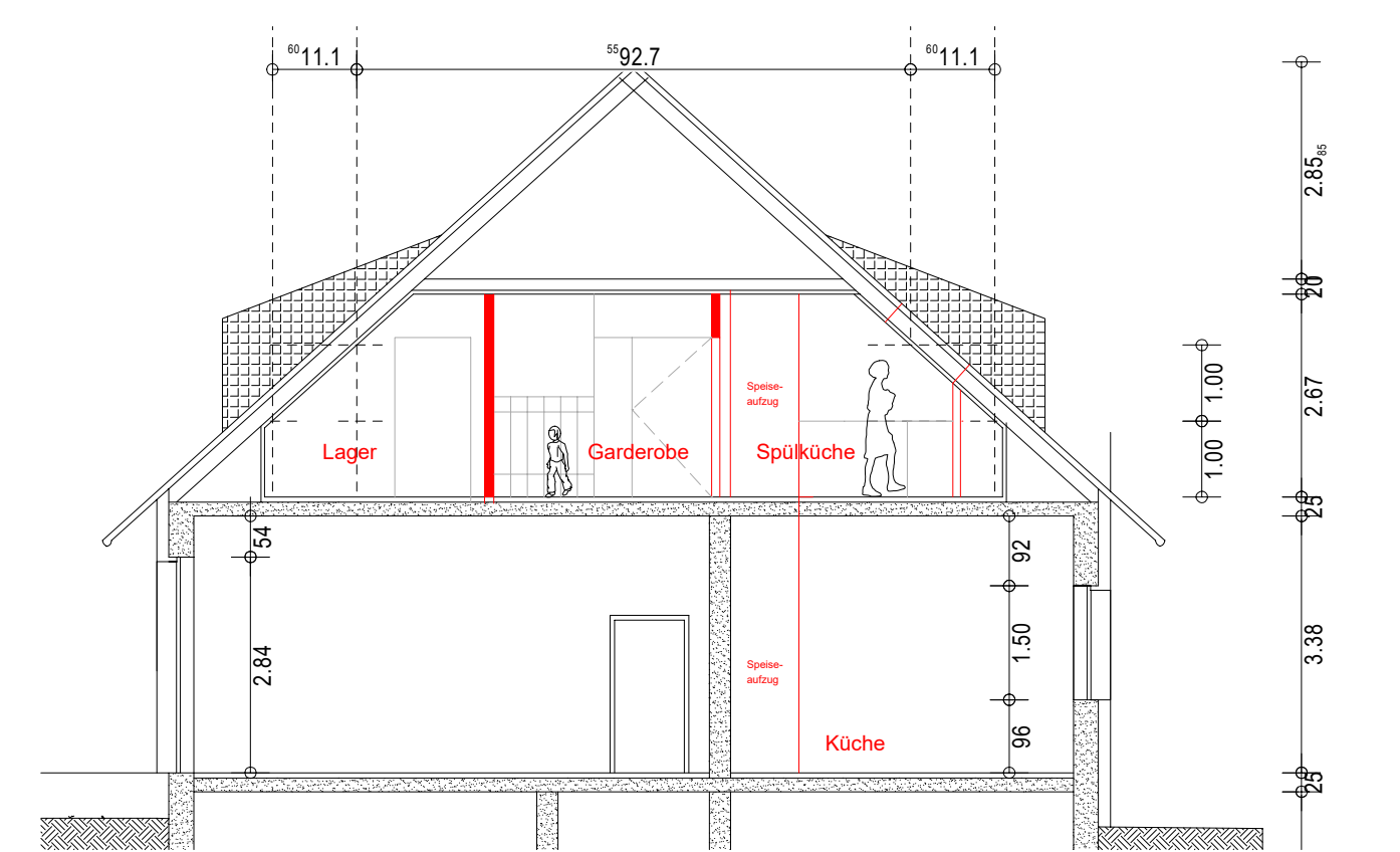
SCHNITT 4 Lager - Garderobe - Spülküche
