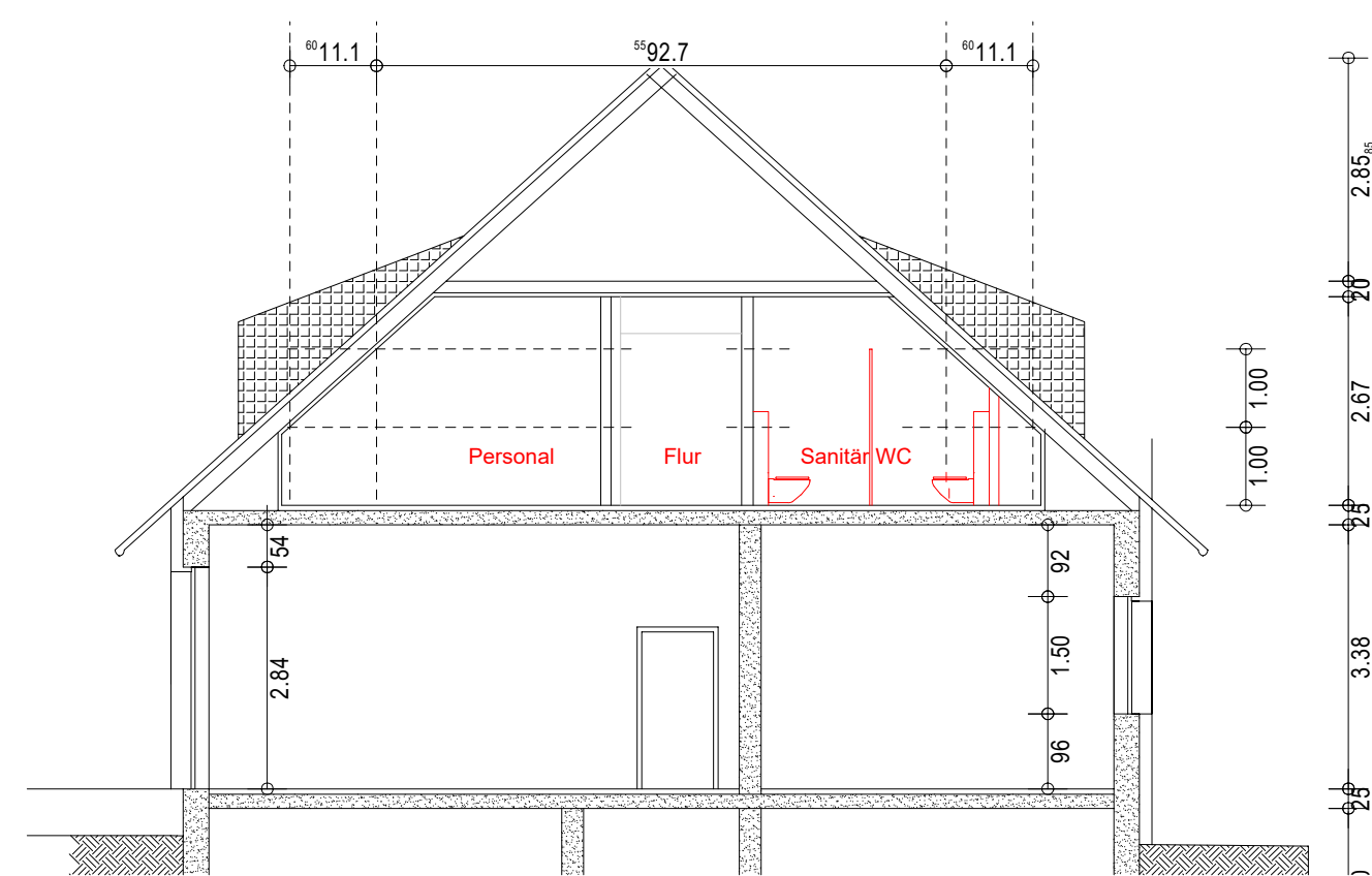
SCHNITT 3 Sanitär/WC - Personal
