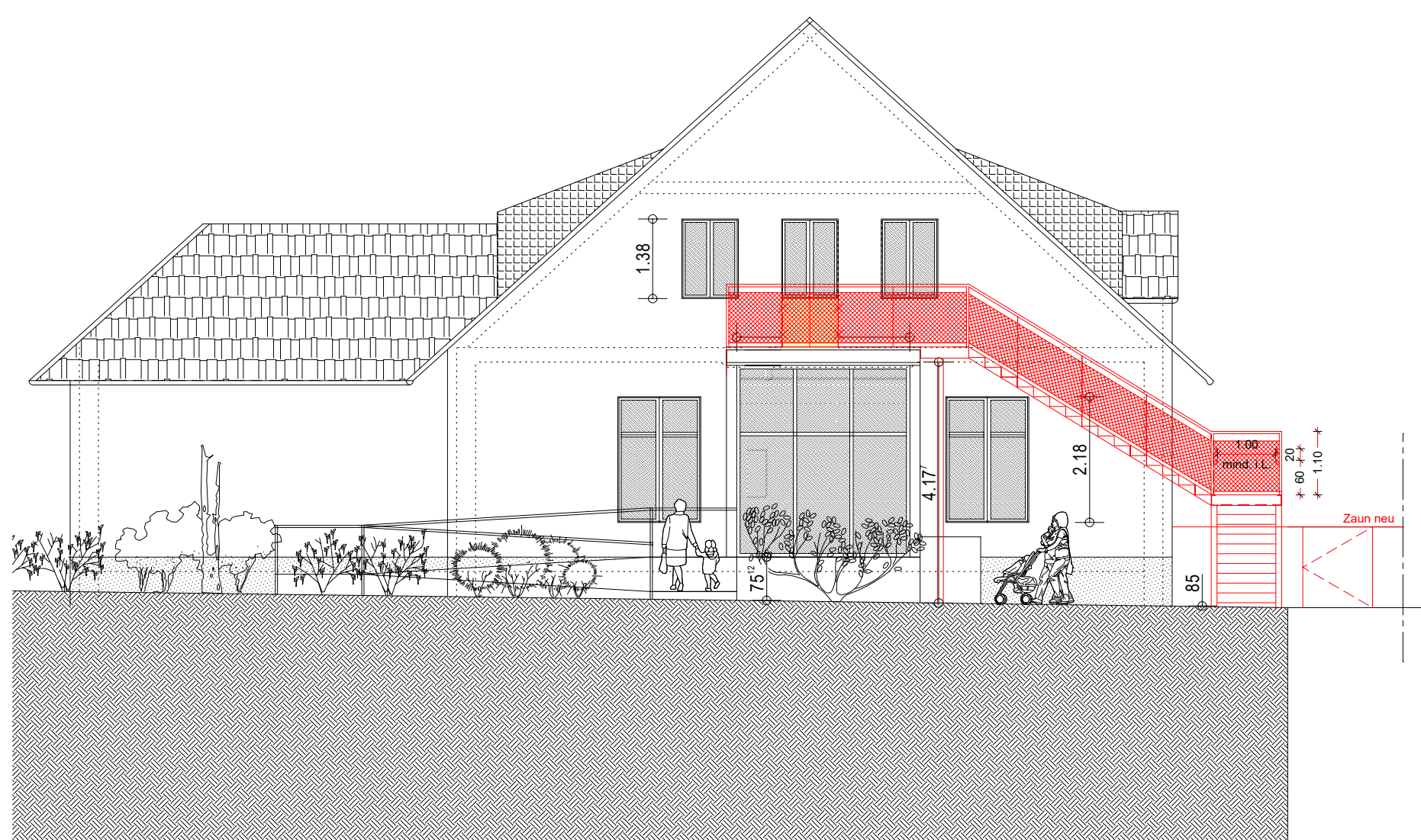
ANSICHT OST
