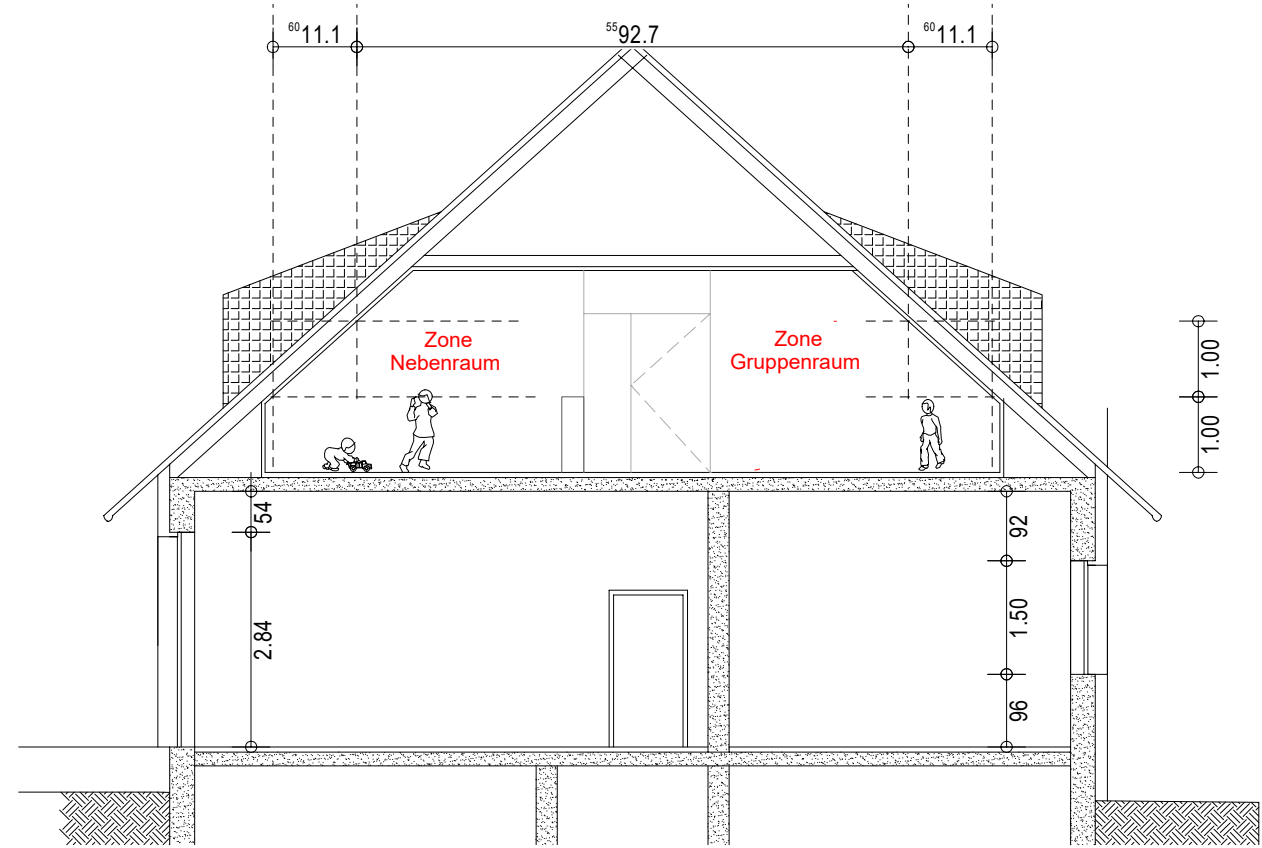
SCHNITT 1 Gruppenraum
