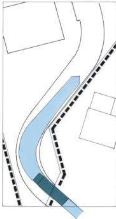
Abbildung 7: Fahrkurve für ein 3-achsiges Müllfahrzeug auf der Haupteinschließung von der Diesterwegstraße.
