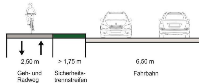
Abb. 2.5.6-3 Kombinierte Geh- und Radweg (außerorts) (gemäß ERA 2010, Kap. 2.2.1)
