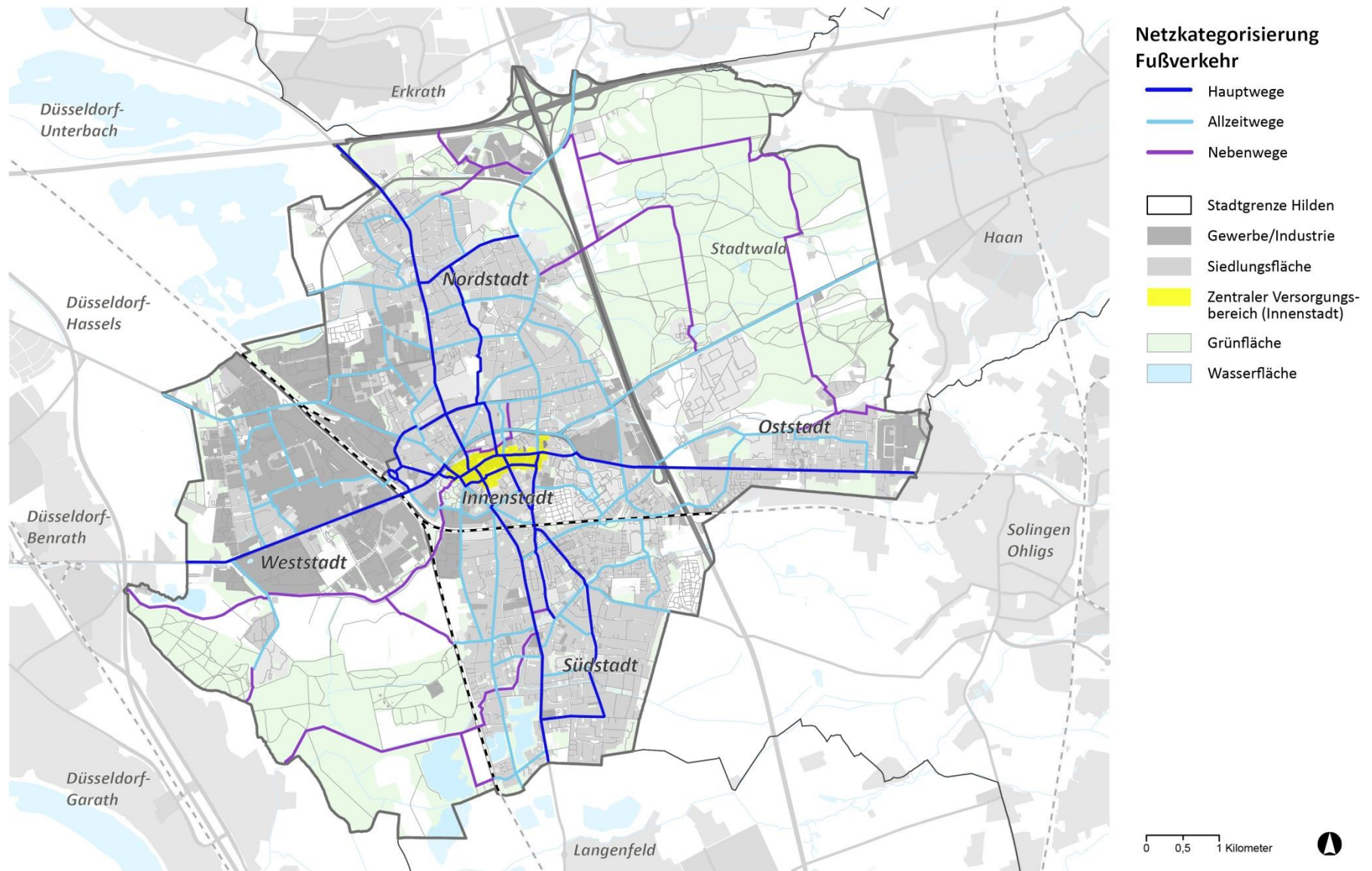
Abb. 2.5.5-1 Netzkategorisierung Fußverkehr
